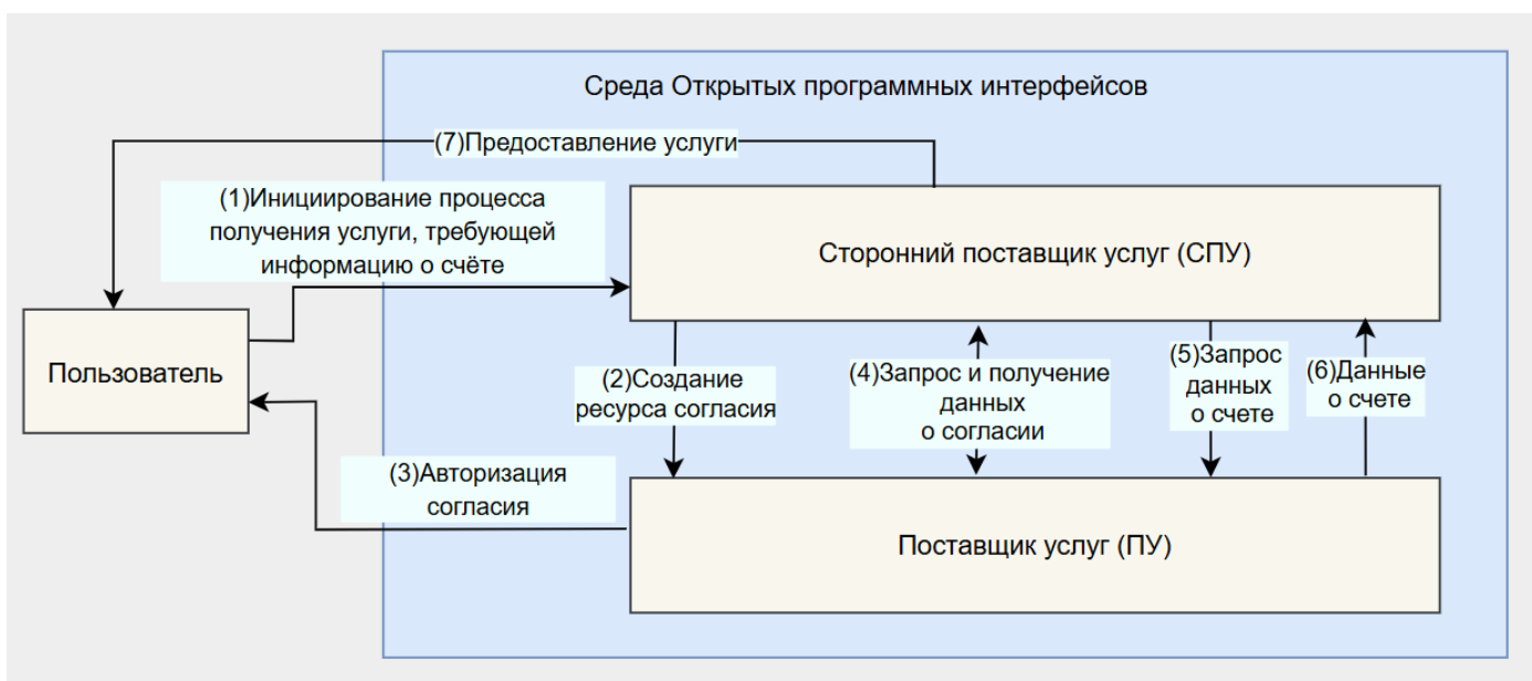
Рисунок 1. Схема взаимодействия Стороннего поставщика услуг (СПУ) и Поставщика услуг (ПУ).
